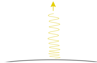
Abbildung 20. Rotverschiebung (schematisch).
