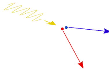
Abbildung 16. Paarerzeugung (schematisch).
