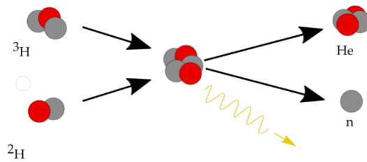
Abbildung 15. Kernfusion (schematisch).
