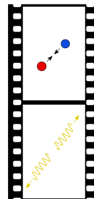
Abbildung 17. Annihilation bei der PET (schematisch).
