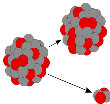
Abbildung 14. Alpha Zerfall (schematisch).
