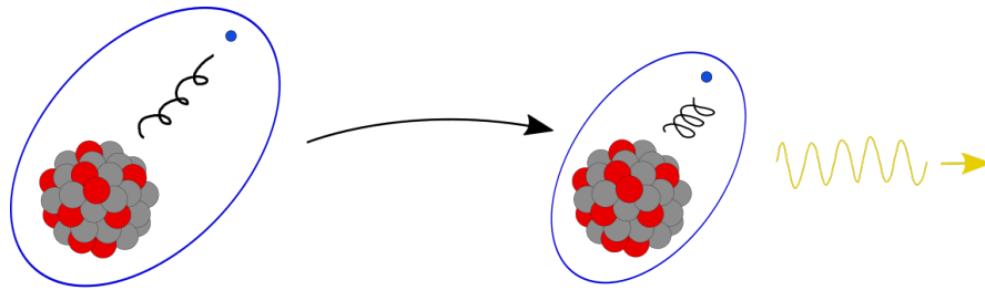
Abbildung 9.3: Darstellung zur Konzeptidee „Elektromagnetische Strahlung ist Feldenergie.“ Durch die Änderung des Abstands von Elektron und Atomkern (Änderung der Wechselwirkung; als Feder dargestellt) strahlt das Atom eine elektromagnetische Welle ab.
